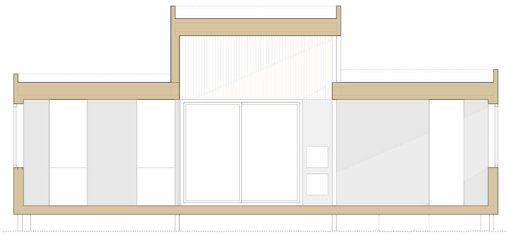
sección aa'
