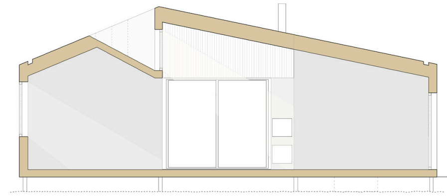
sección aa'
